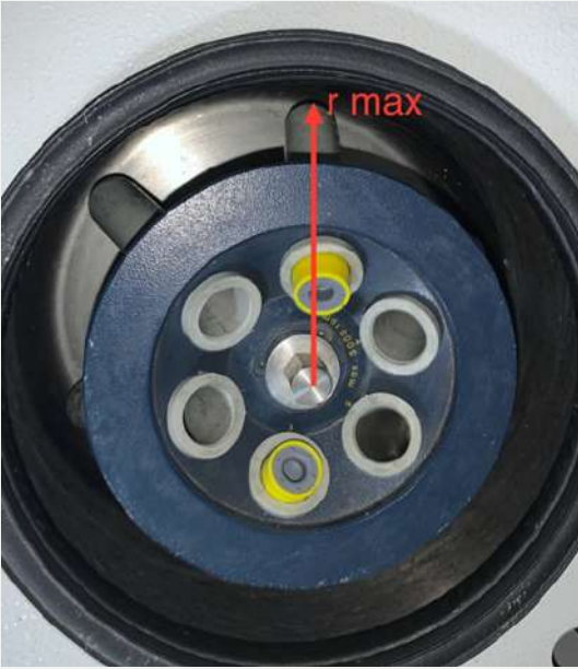
Şekil 1 “Açılı rotor” için r max ölçümü örneği
